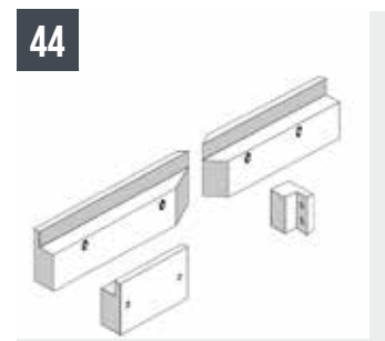
44 TIGER 352 MA/SXevo TIGER 372 SXevo Série de mâchoires pour menuiseries métalliques H 50
