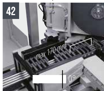
42 TIGER 352 NC 5.0 - Série de mâchoires à peigne 70x70 mm max. pour réduire la chute du matériau à couper
