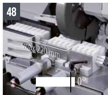
48 COBRA 352 NC 5.0 - Série de mâchoires à peigne 70x70 mm max. pour réduire la chute du matériau à couper
