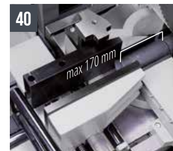
40 TIGER 352 NC 5.0 Étau spécial pour réduire la chute
