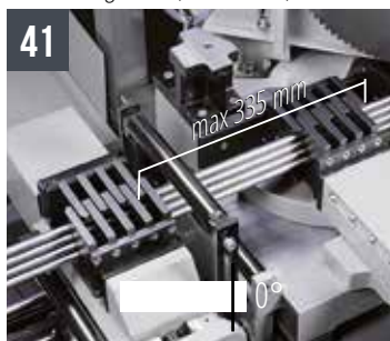
41 TIGER 352 NC 5.0 max 70x70 Série de mâchoires à peigne
