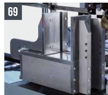
69 SHARK 230 NC HS 5.0 étau de coupe à double serrage
