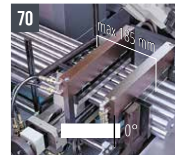
70 SHARK 331 NC 5.0 spider - Étaux verticaux hydrauliques pour coupe en paquets (max 320x150 mm)
